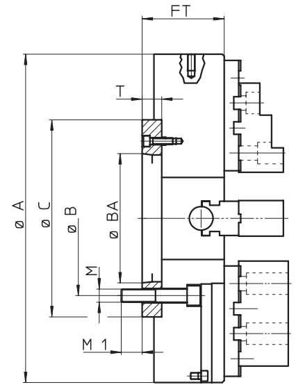
Tipo 1 montaggio ISO-A diretto direct ISO-A mounting
